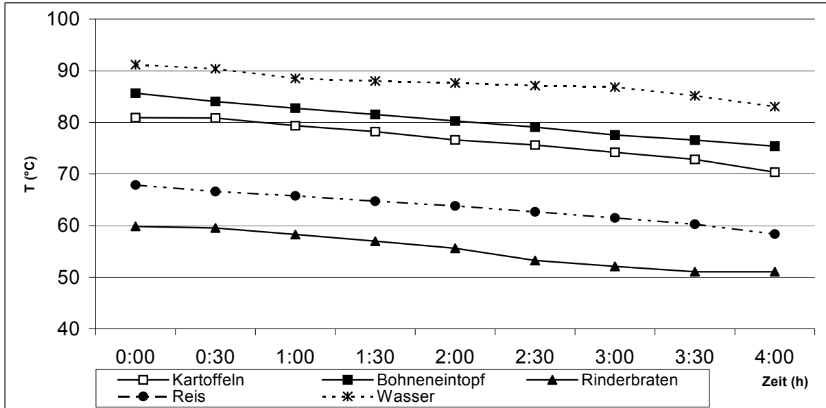
Abbildung 2: Temperaturverläufe von Wasser, Bohneneintopf, Kartoffeln, Reis und Rinderbraten in einem Transportbehälter mit einer maximalen Füllmenge von 26 Litern
